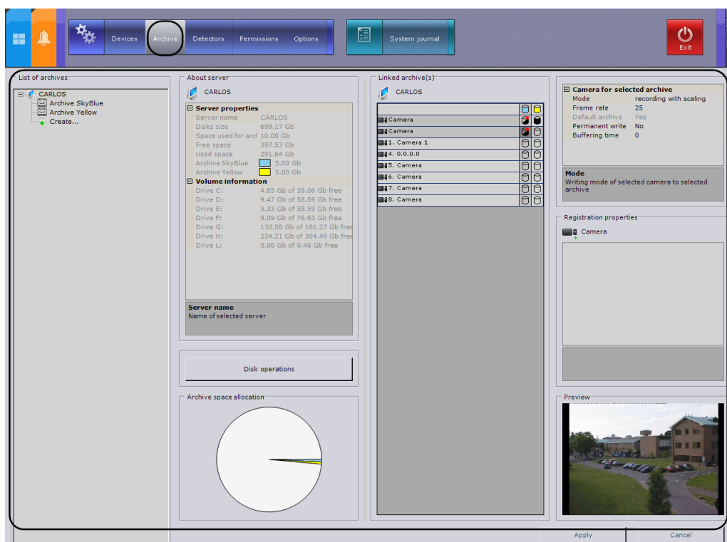
Fig. 6.5—1 The Archive tab
