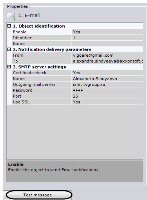
Fig. 6.3—27 Checking E-mail notification
