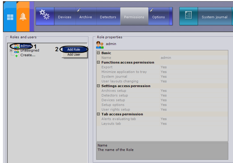
Fig. 6.10—1 Adding a role
