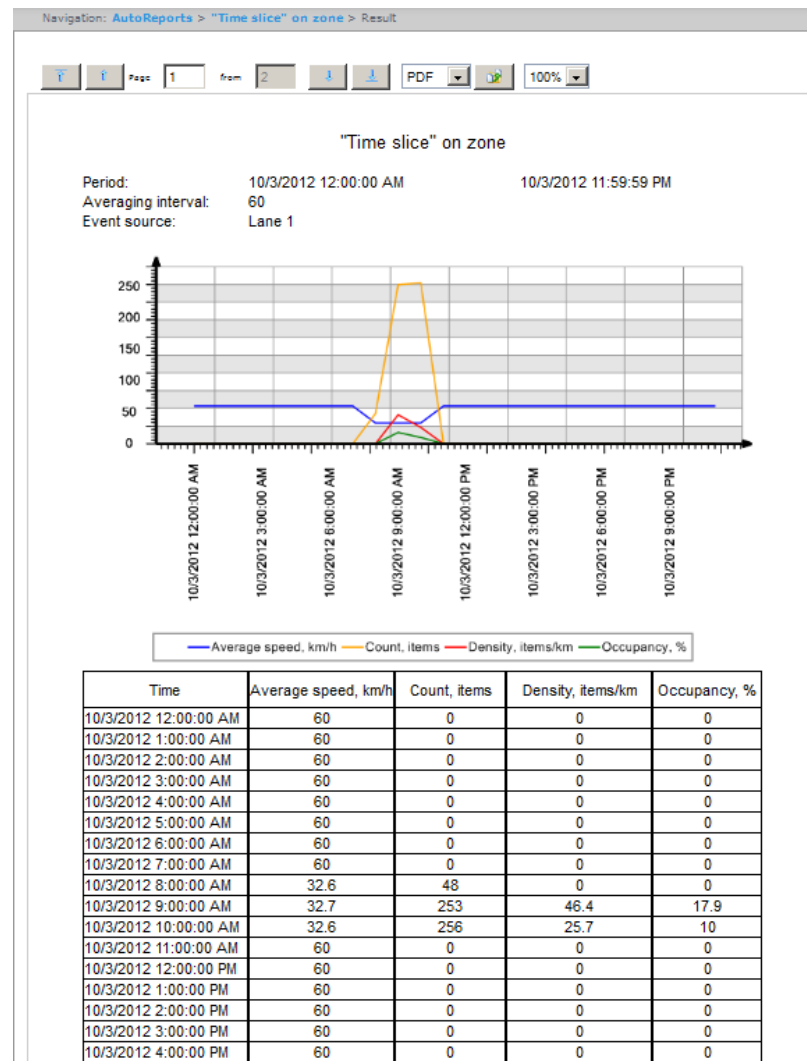
Figure 8.4—6 Example of «Time slice» on zone
