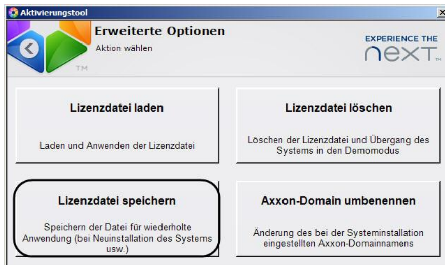
Abb. 5.3—2 Fenster der erweiterten Optionen
