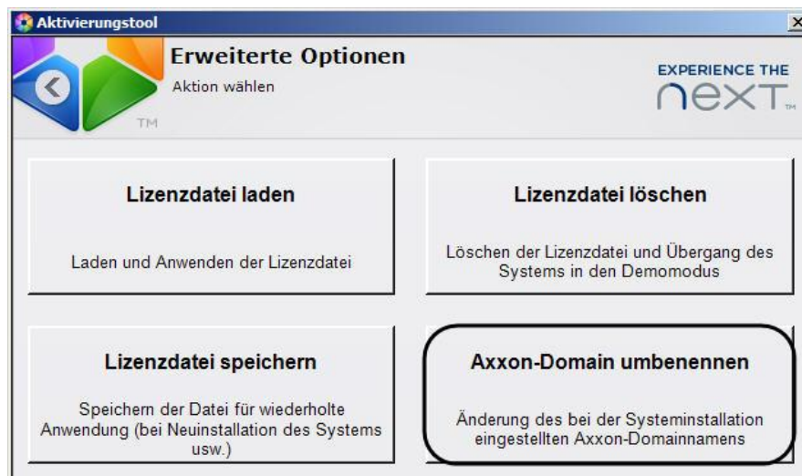
Abb. 5.4—2 Fenster der erweiterten Optionen
