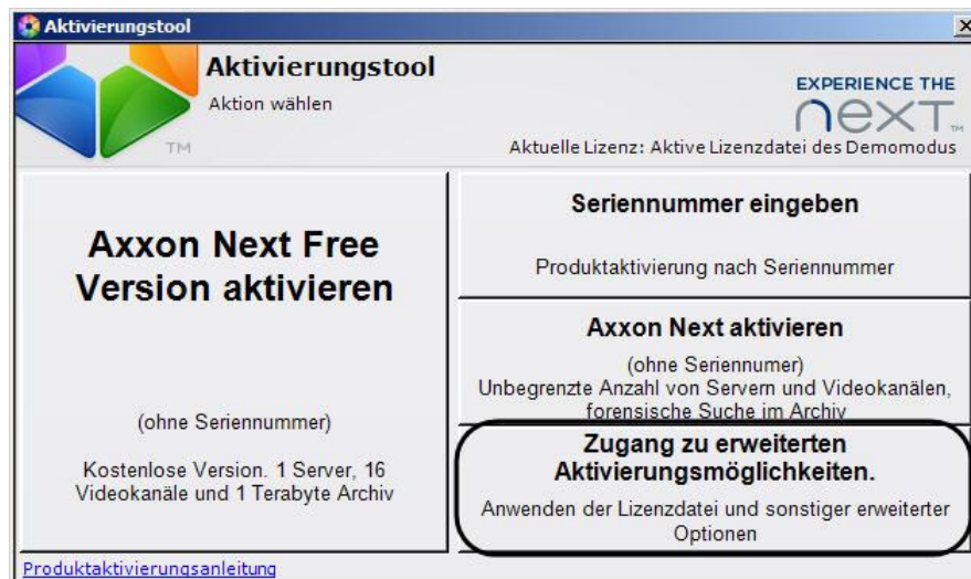
Abb. 5.1—1 Übergang zu zusätzlichen Optionen
